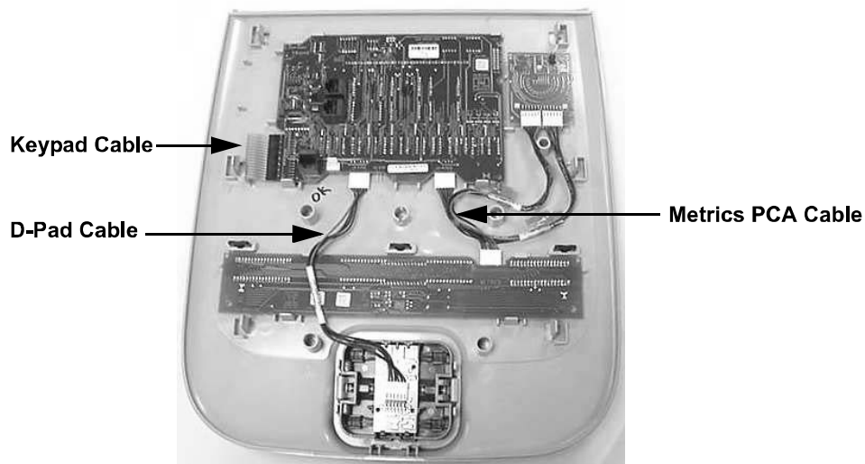
Diagram 6.1 - Upper PCA & Keypad
