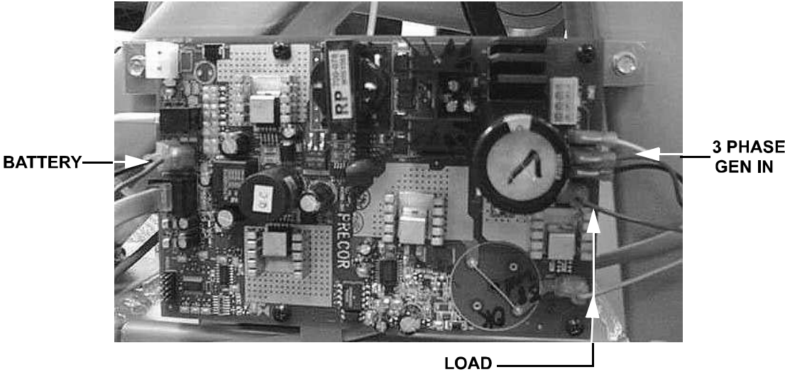
Diagram 5.1 - Lower PCA
