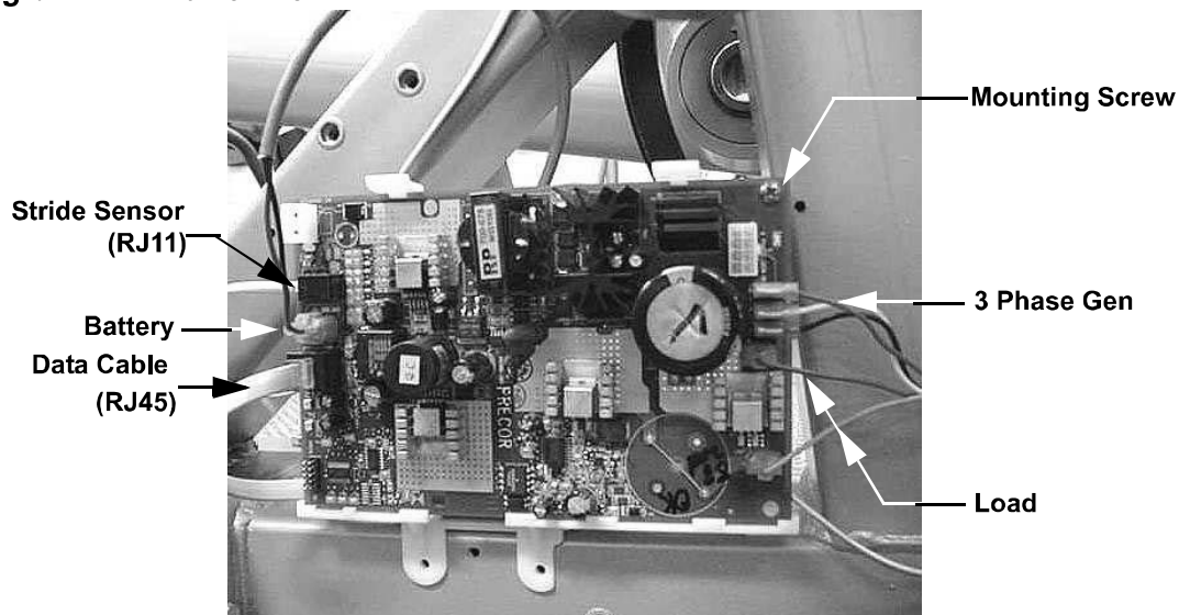
Diagram 7.2 - Lower PCA
